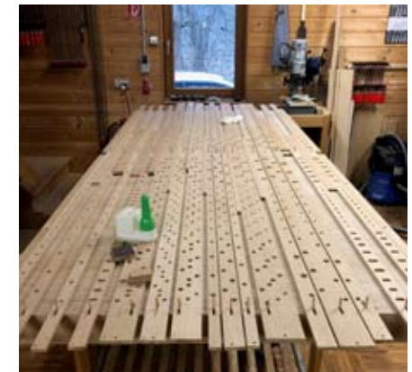
Schleifen der Chororgel in der Werkstatt. Später werden sie mit den Registerzügen bewegt. (Foto: Friedrich Lieb)
